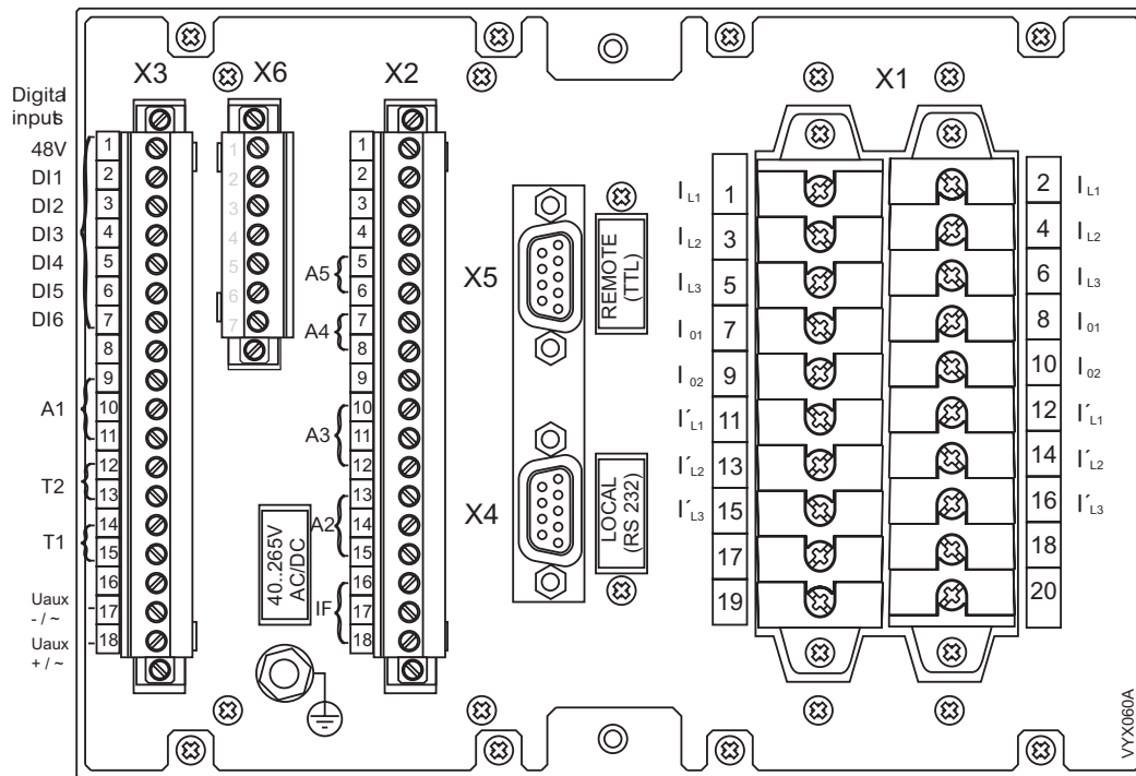
VAMP265rearPanel
